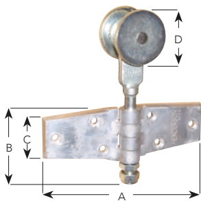
MELLANHÄNGRULLE 62
