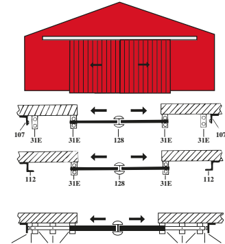
DUBBEL SKJUTPORT
