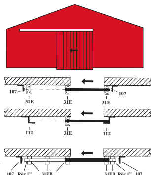
ENKEL SKJUTPORT
