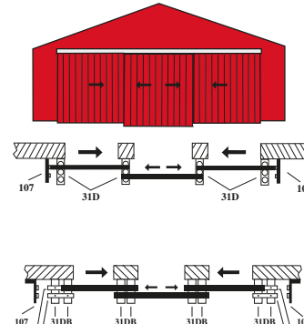
OMLOTTGÅENDE SKJUTPORT
