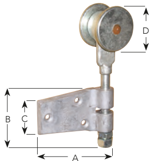
ÄNDHÄNGRULLE 63
